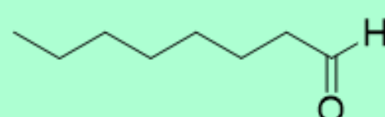
1-Octanal
