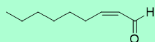
(Z)-2-Nonenal
