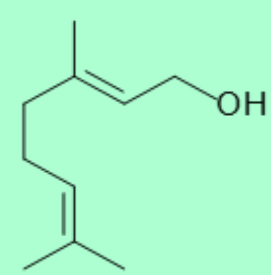
Geraniol
