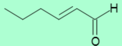
(2E)-hexenal
